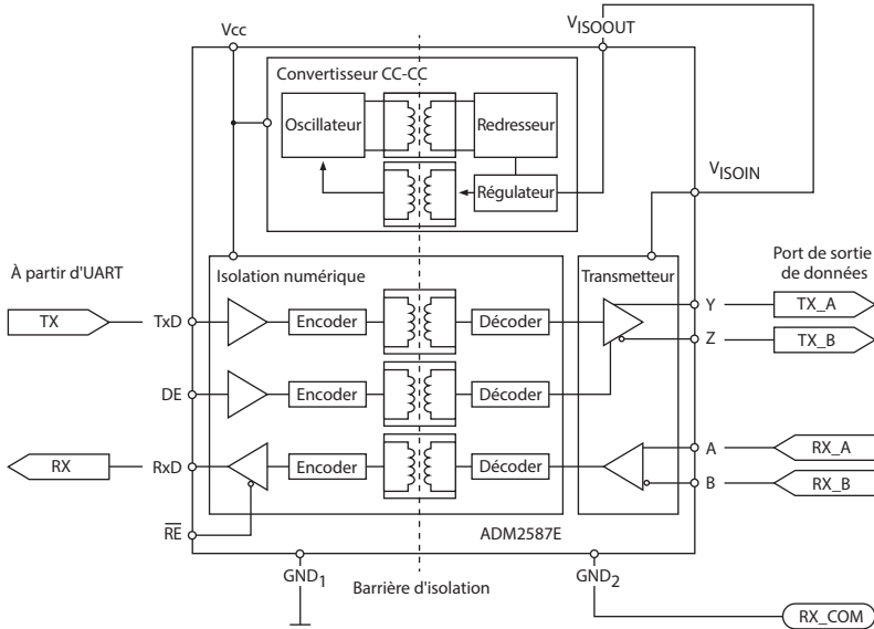
Figure 30 Schéma du port de sortie de données
