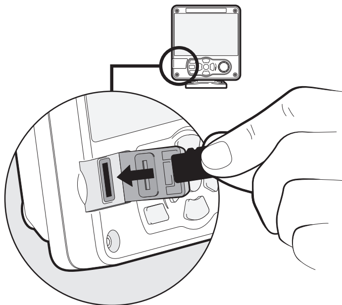
Figure 26 Port pour carte Micro SD
