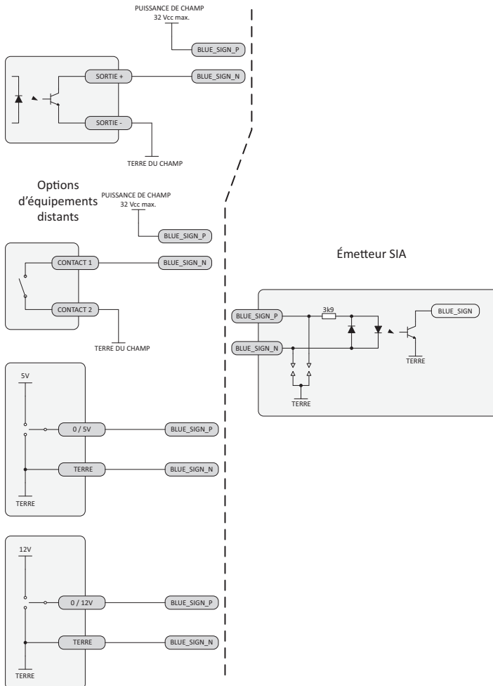
Figure 28 Options de raccordement de l'interface Signal bleu
