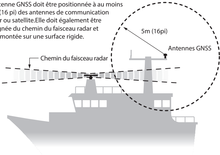
Figure 7 Emplacement de l'antenne GNSS
