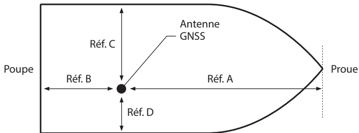
Figure 36 Position de l'antenne GNSS
