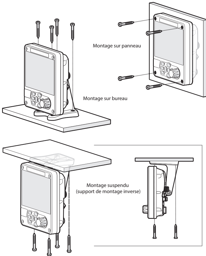
Figure 4 Installation de l'émetteur SIA
