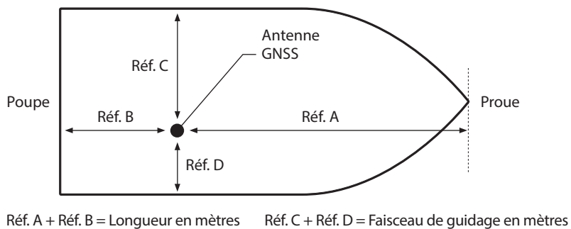
Figure 23 Mesure des dimensions du bateau
