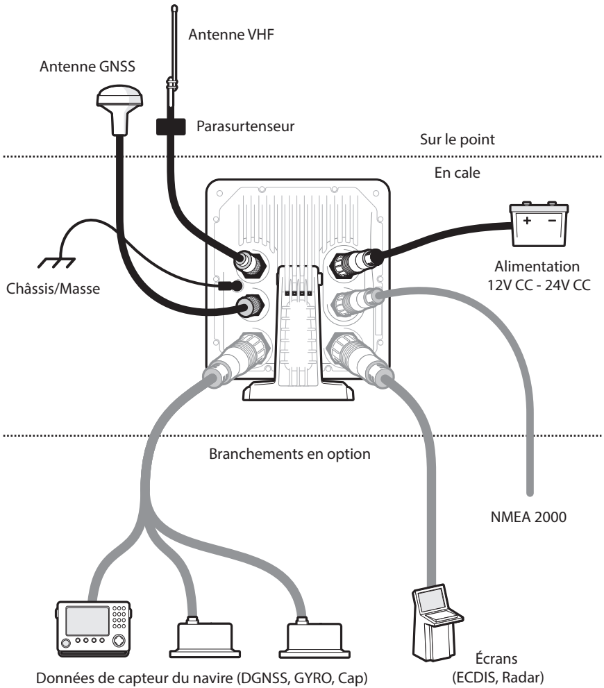
Figure 3 Connexion type de l'émetteur SIA
