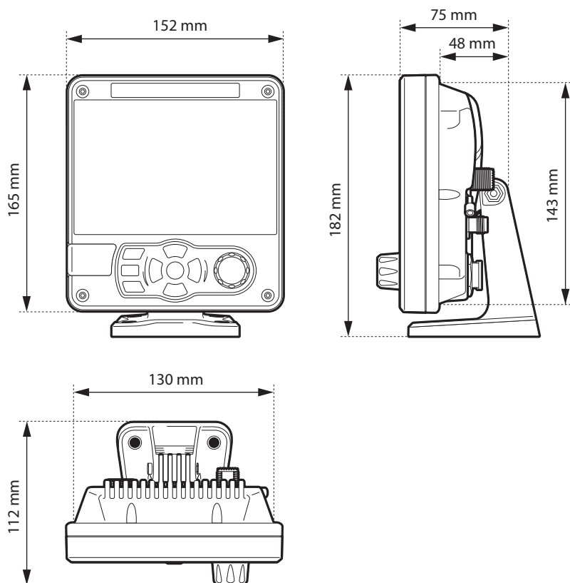
Figure 31 Dimensions de l'émetteur SIA
