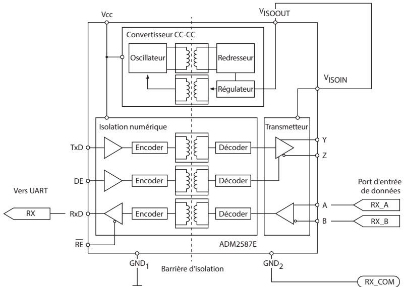
Figure 29 Schéma du port d'entrée
