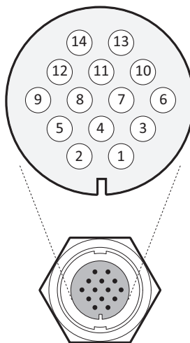
Figure 12 Connexion des câbles du connecteur 14 broches
