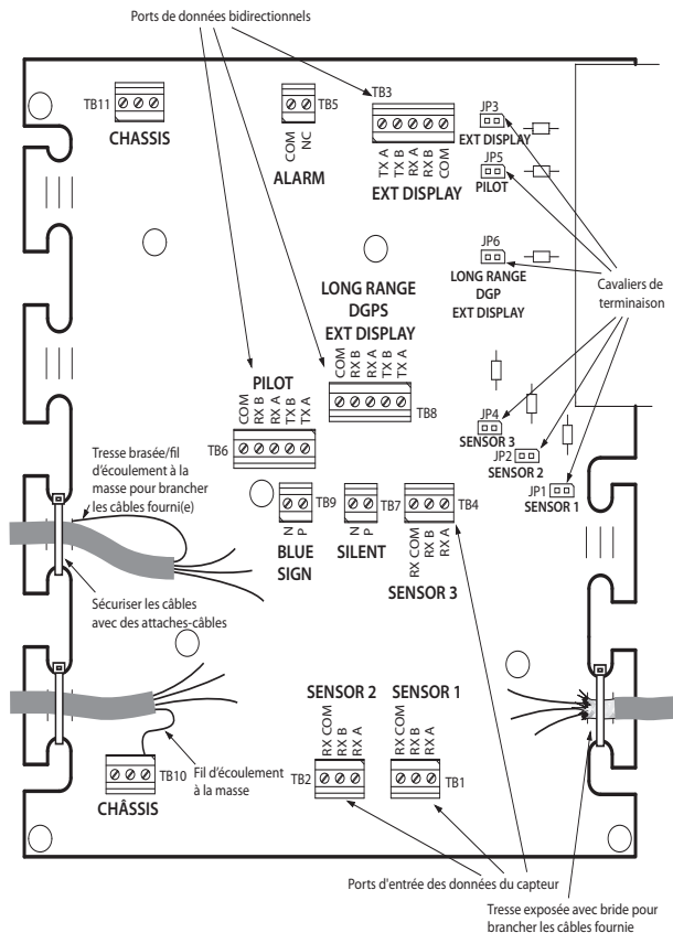
Figure 34 Raccordements de la boîte de connexion
