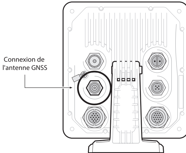
Figure 7 Emplacement de l'antenne GNSS
