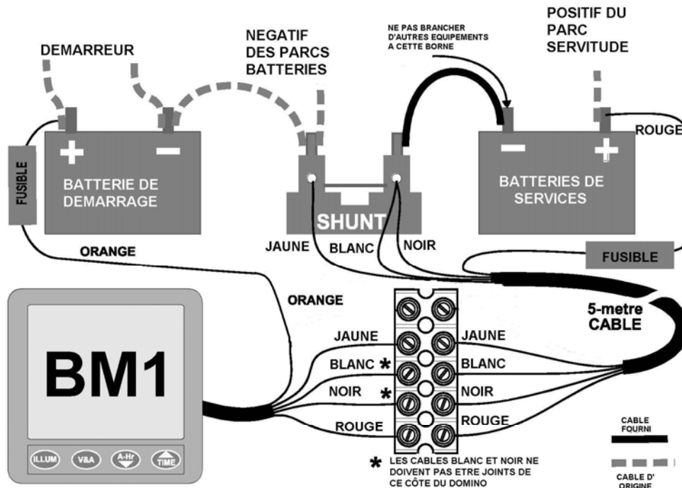
Figure 2 : Plan de câblage batteries de service + démarrage
